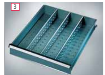
3 Fachschiene, Stahlblech verzinkt. Am Schubfachboden verschraubbar. Für Blendenhöhe mm
